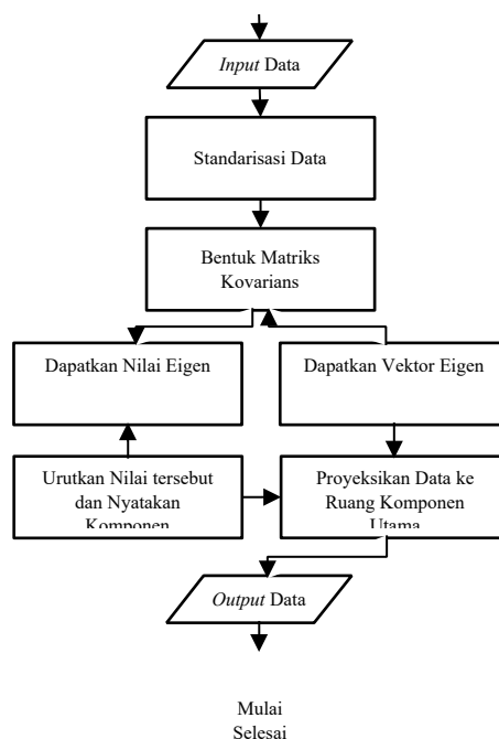
Gambar 1. Flowchart metode PCA secara umum
