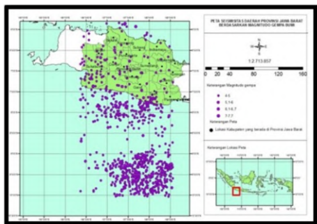
Gambar 2. Peta seismisitas berdasarkan magnitudo gempa bumi.
