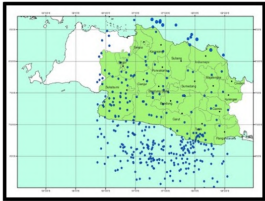
Gambar 5. Penyebaran peta seismisitas berdasarkan kedalaman gempa bumi.
