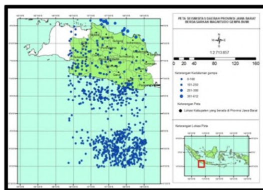
Gambar 4. Peta seismisitas berdasarkan kedalaman gempa bumi.
